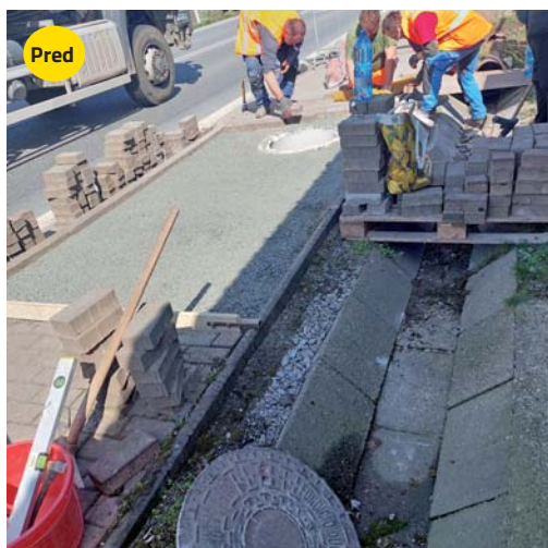
Rekonštrukcia chodníka v obci Proč – výška NFP – 38 553,92 €
